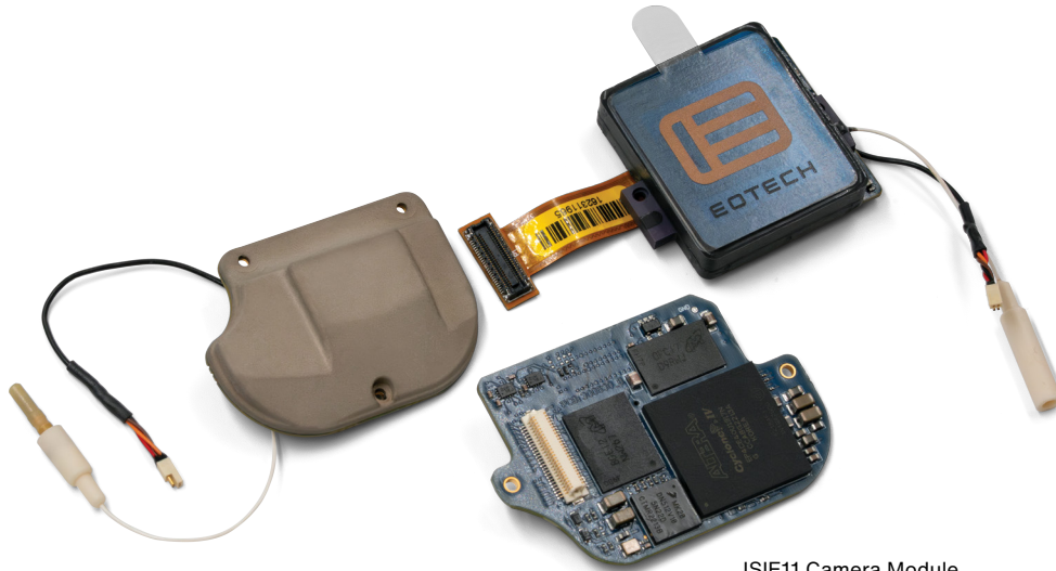
ISIE11 Camera Module
